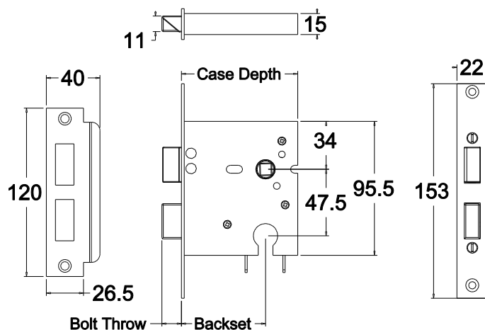
JMC60
