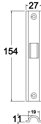
Astragal Striker
