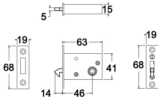
JSP1, JSL2
