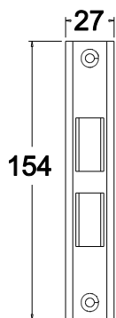
Astragal Striker
